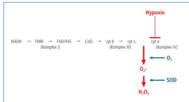
Abb. 7: Schema der Elektronenübertragung bei der Zellatmung. Sauerstoffmangel führt dazu, dass der Elektronentransport von Komplex III auf Komplex IV der Atmungskette unterbrochen ist. Die aufgelaufenen Elektronen werden auf Sauerstoff übertragen, was zur Bildung von Superoxid-Anionen führt.
