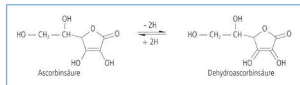
Abb. 13: Ascorbinsäure
