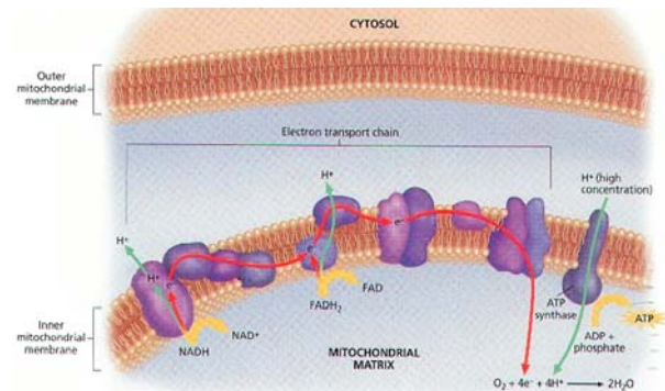
Abb. 6: Elektronentransportkette in der inneren Membran der Mitochondrien. Am Ende der Reaktionsschritte (Zellatmung) steht die Bildung von Wasser. Rund 98% des Sauerstoffs der Zelle werden auf diesem Wege zu Wasser reduziert. 2% des Sauerstoffs werden zu reaktiven Sauerstoffspezies umgewandelt.
