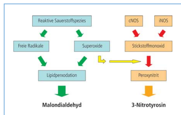
Abb. 5: Reaktionswege zur Bildung freier Radikale und ihrer Indikatormoleküle Malondialdehyd und 3-Nitrotyrosin. iNOS: induzierbare NO-Synthase, cNOS: konstitutive NO-Synthase
