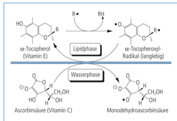
Abb. 3: Wirkmechanismen der Antioxidantien Tocopherol (Vitamin E) und Ascorbinsäure (Vitamin C)
