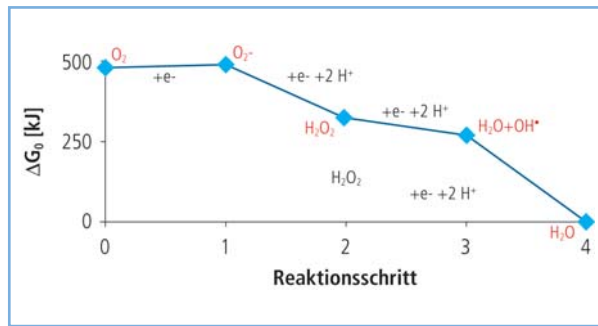
Abb. 4: Reaktionskette, die zur Bildung reaktiver Sauerstoffspezies führt. Lediglich der erste Schritt dieser Kette, die Bildung des Superoxid-Anions bedarf der Zufuhr von Energie. Alle anderen Reaktionen laufen spontan ab. Die übertragenen Elektronen stammen von Metallionen.
